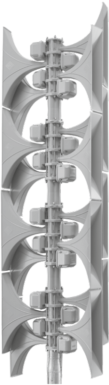
SIRENENKOPF aus selbsttragenden Sirenenhörnern in modularem Aufbau.
