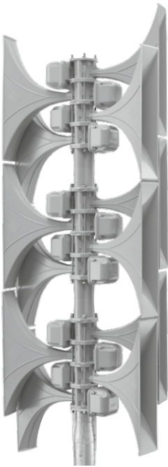
SIRENENKOPF aus selbsttragenden Sirenenhörnern in modularem Aufbau.
