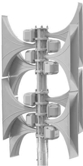
SIRENENKOPF aus selbsttragenden Sirenenhörnern in modularem Aufbau.
