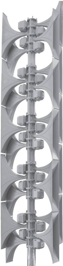
SIRENENKOPF aus selbsttragenden Sirenenhörnern in modularem Aufbau. 360° omnidirektionale Schallausbreitung durch Spalteffekt.
